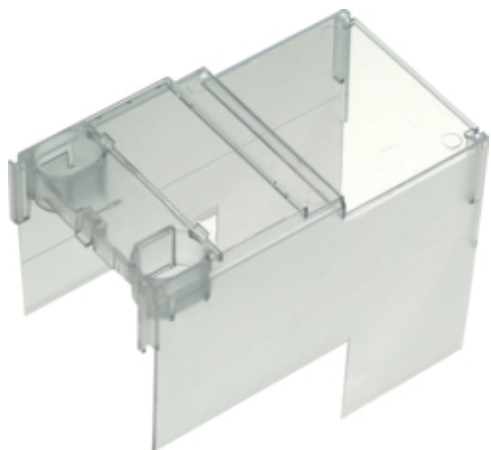
Capac protectie lung, NH1-3/185 mm
